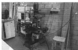
DESCRIÇÃO: FRESADORA, MARCA CARDOSO FC-30, 1 UNIDADE.
