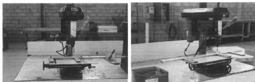
DESCRIÇÃO: FURADEIRA DE BANCADA, MARCA MOTO MIL, MOD. FB160, 2 UNIDADES.
